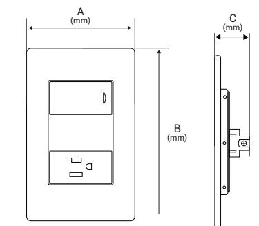
Placa con botón timbre JTL-E7513: 15A 127V~60Hz
