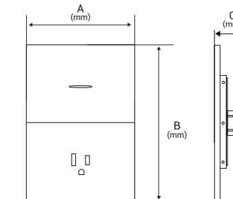
Placa con botón timbre JTL-G7713: 10A 127V~60Hz
